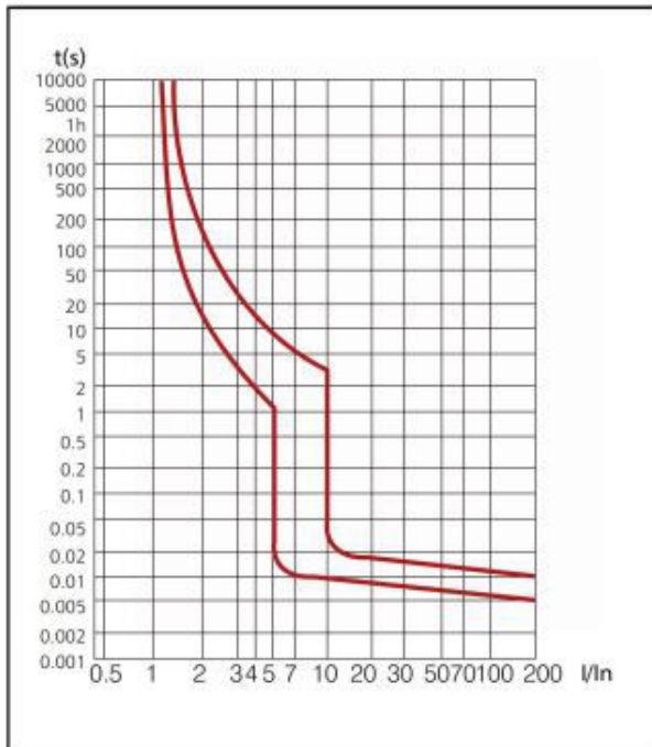
Kennlinie C
